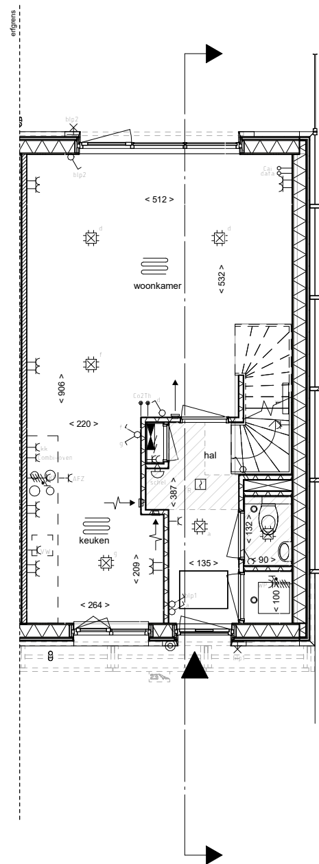
begane grond
