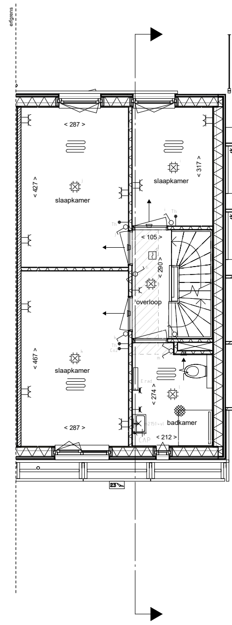
eerste verdieping
