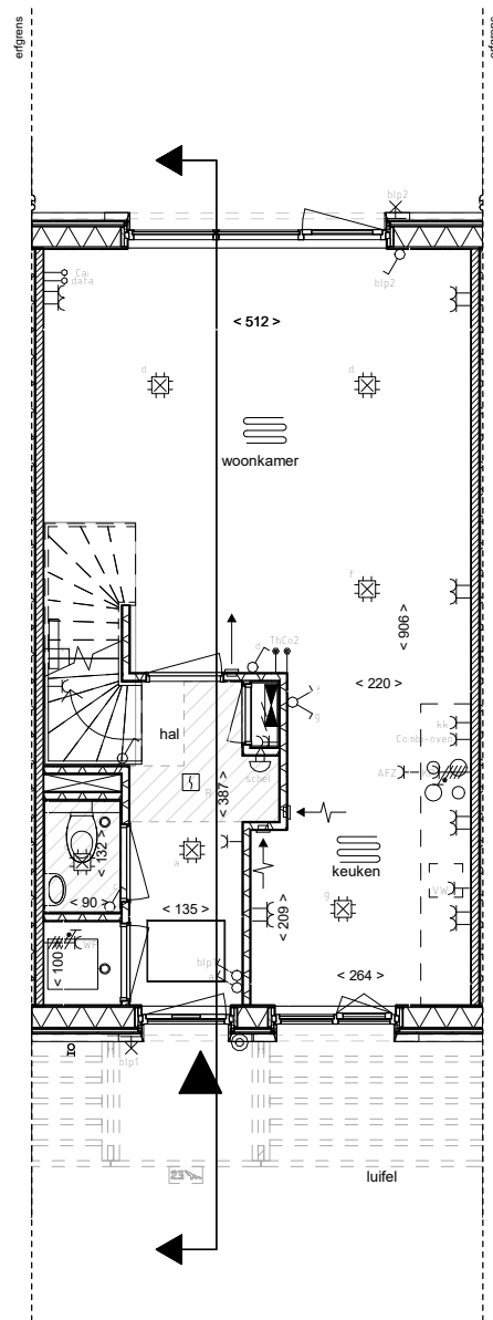
begane grond
