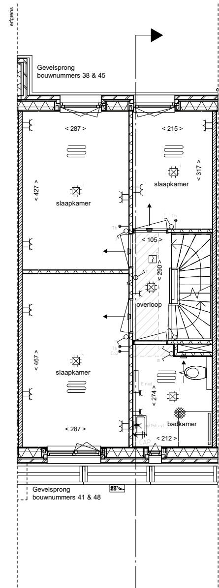
eerste verdieping
