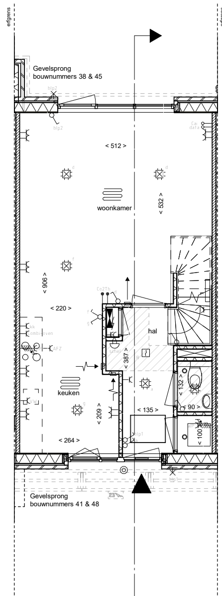
begane grond
