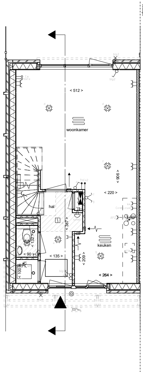
begane grond
