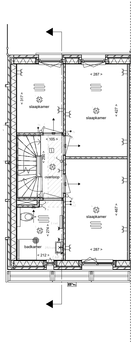
eerste verdieping
